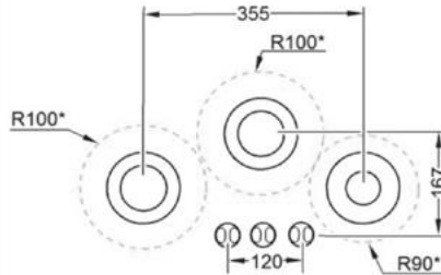
Aufbau der Brenneranordnung auf der Grundplatte des Modells Topline 167: 1 x 1, 0 kW: 2 x 1,5 kW
