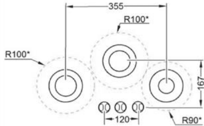
Aufbau der Brenneranordnung auf der Grundplatte des Modells Topline 167: 1 x 1, 0 kW: 2 x 1,5 kW
